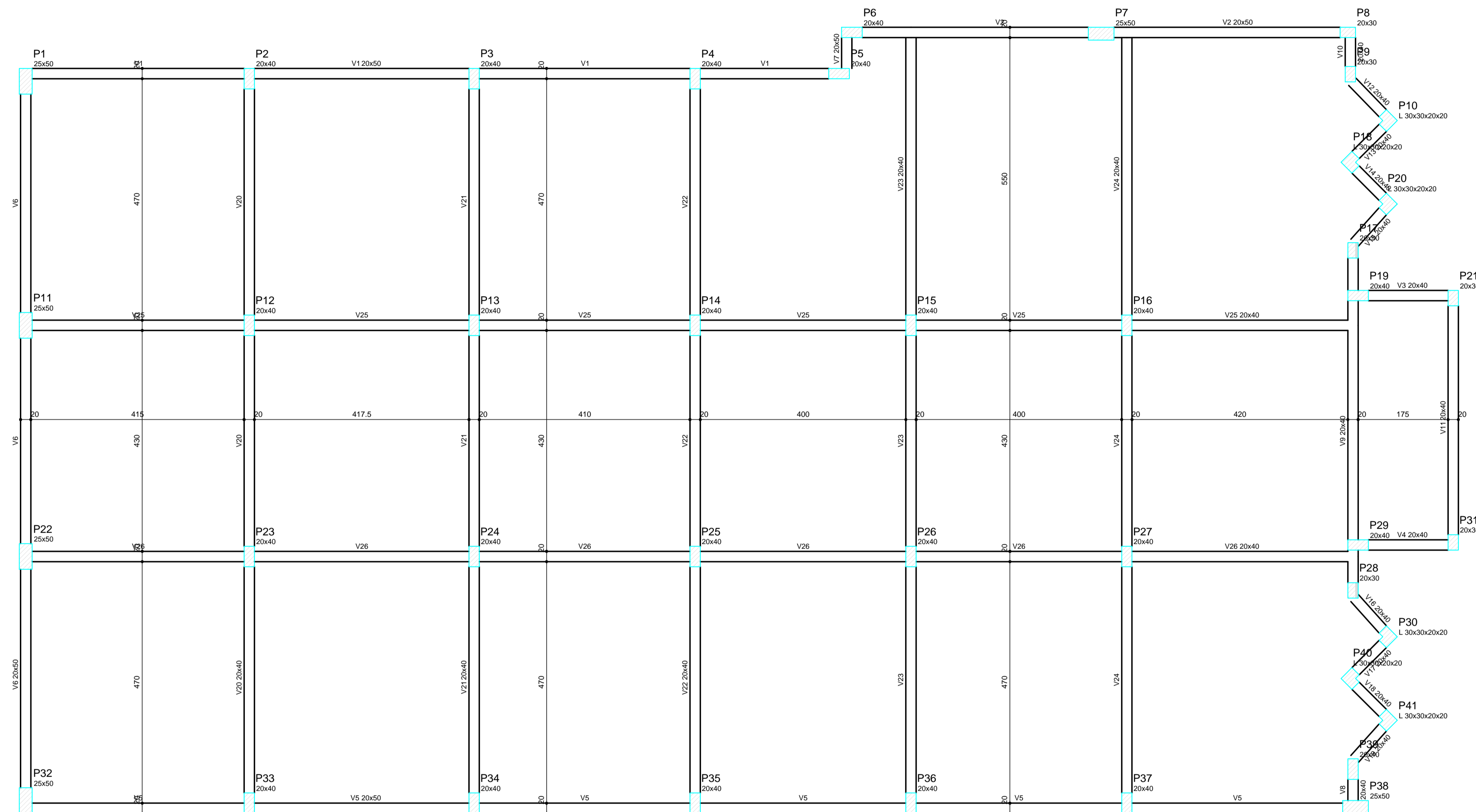
Forma do pavimento BALDRAME escala 1:50
